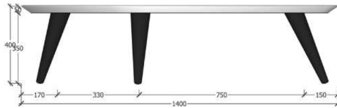
TAMPAK DEPAN
