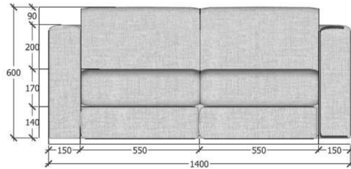
TAMPAK DEPAN
