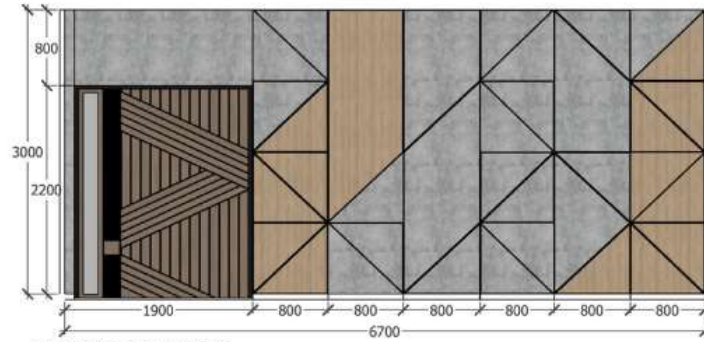
TAMPAK BELAKANG
