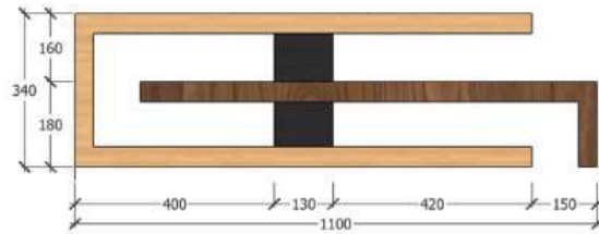
TAMPAK ATAS
