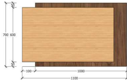
TAMPAK ATAS
