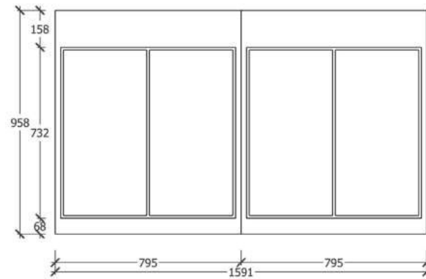
TAMPAK ATAS
