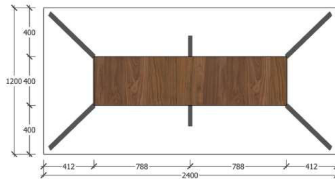
TAMPAK ATAS
