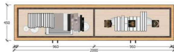
TAMPAK ATAS
