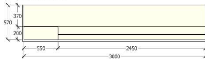
TAMPAK ATAS
