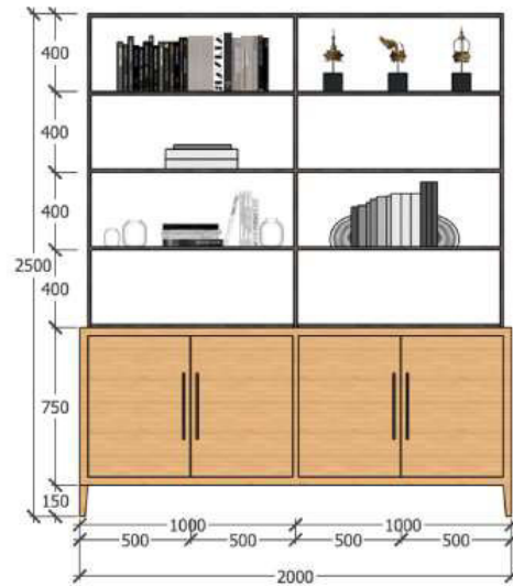
TAMPAK DEPAN
