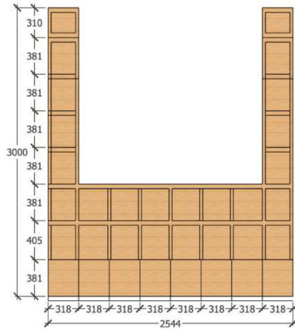
TAMPAK ATAS
