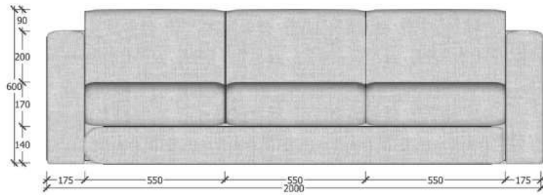
TAMPAK DEPAN
