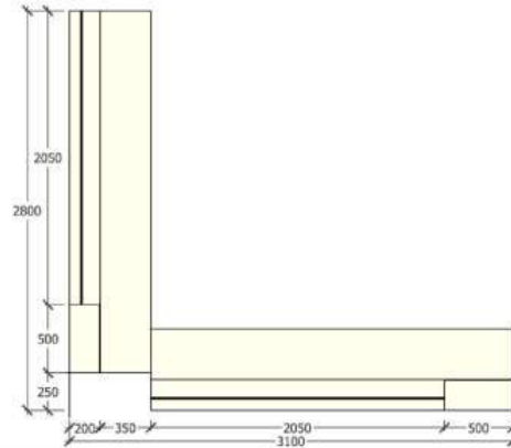
TAMPAK ATAS
