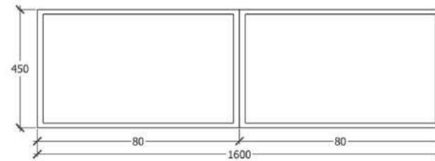
TAMPAK ATAS
