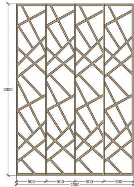
TAMPAK DEPAN
